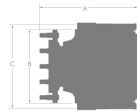
Spindle Flange Output
